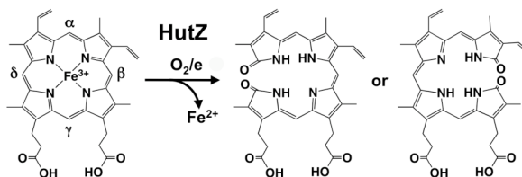
図2: HutZによるヘムの分解
